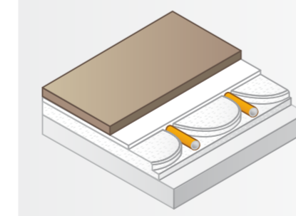
Variomodul-Rohr 11,6 x 1,5 / Alu 0,20
